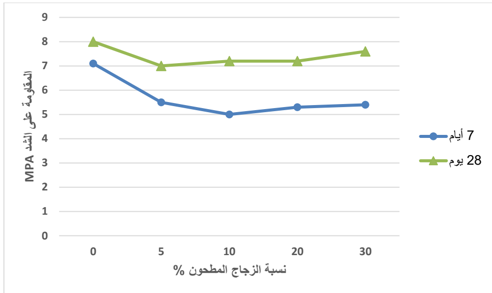
الشكل (5): المقاومة على الشد بالانعطاف
