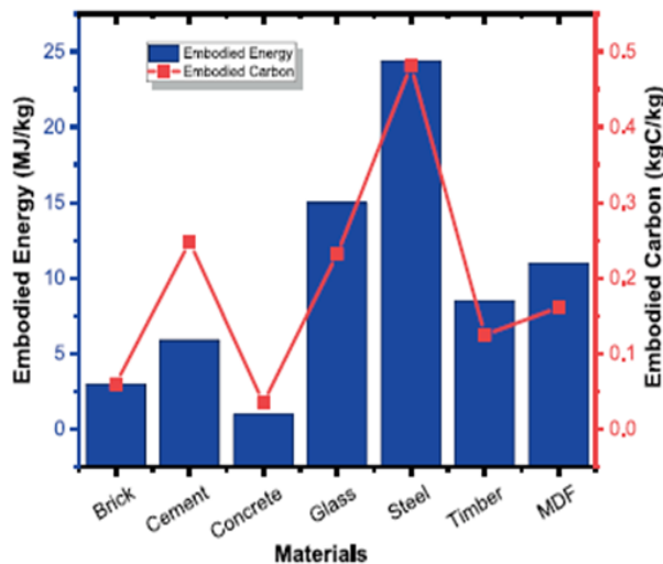
الشكل (1): الطاقة المستهلكة والكربون المنتج لمواد البناء [7]
