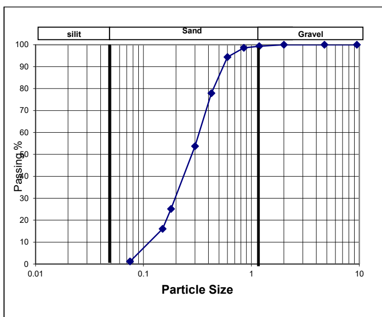
الشكل (2): منحنى التحليل الحبيبي للرمل المستخدم في الخلطة
