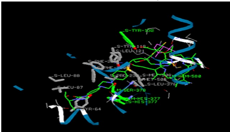
الشكل (6): ارتباط مركب BETANIDIN ضمن الجيب الفعال للإنزيم FSA5 (اللون البنفسجي) والمركب العياري X2N (اللون الأخضر) بالإضافة إلى وجود الروابط الهيدروجينية (باللون الأخضر) وروابط فان دير فالس (باللون الرمادي).
