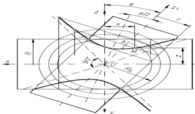
الشكل (3): تقاطع أسطوانتين دورانيتين محوراهما غير متعامدين R > r
