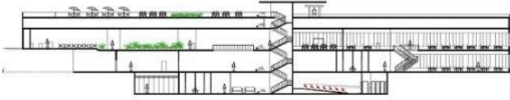
المقطع AA
